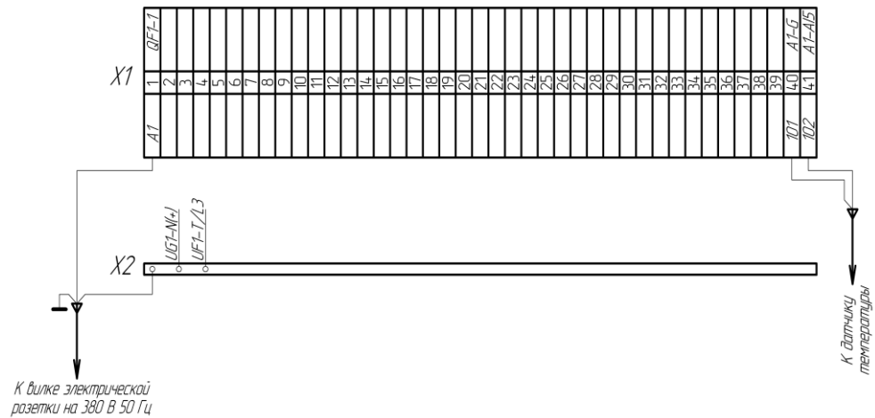
Рис. 2. Схема электрическая монтажная
