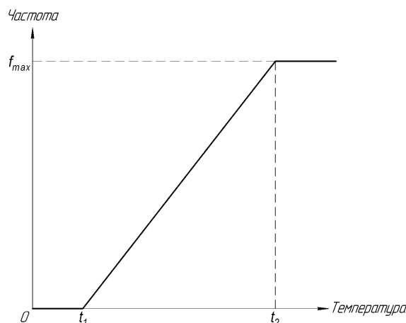
Рис. 4. Зависимость частоты, выдаваемой частотным преобразователем на двигатель, от температуры
