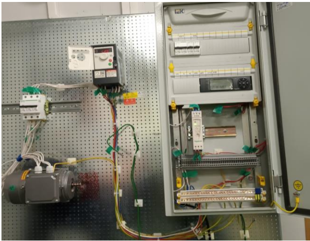
Рис. 3. Внешний вид стенда на этапе сборки
