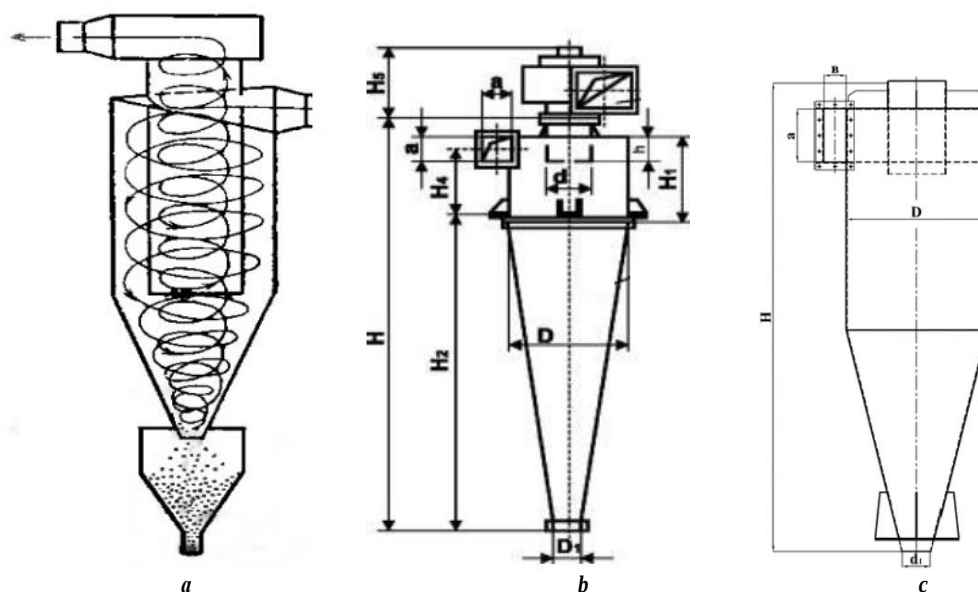
Рис. 2. Конструктивное оформление циклонов: a) ЦН – циклон НИИОГАЗа; б) УЦ – универсальный циклон; в) СЦН – спиральный циклон НИИОГАЗа
