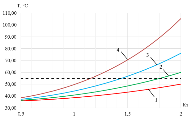
Рис. 2. Зависимости температуры нагрева контактов автоматического выключателя ВА04
