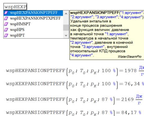
Рис. 9. Расчет процесса расширения пара в турбине
