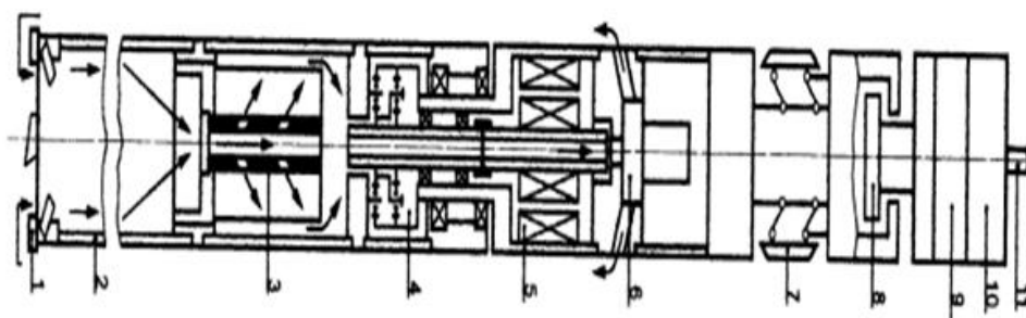
Рис. 2 – Электромеханический бур КЭМС-132: 1 - буровая головка, 2 - колонковый бур, 3 - камера с фильтром для шлама, 4 - редуктор, 5 - приводной электродвигатель, 6 - насос, 7 - противомоментная система, 8 - ударный блок, 9 - электрокамера, 10 - скоба подвеса троса, 11 – трос
